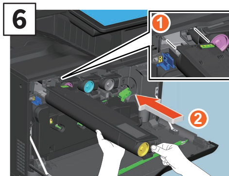
6 Lijn de nieuwe tonercartridge uit met de geleider. Plaats het ter hoogte van de zwarte lijn.
