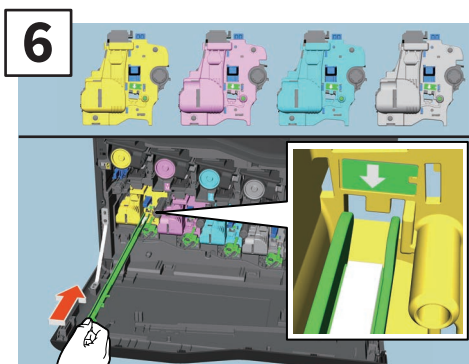
6 Steek de reiniger door het onderhoudsgat van de developer onder de pijl tot tegen het einde.
