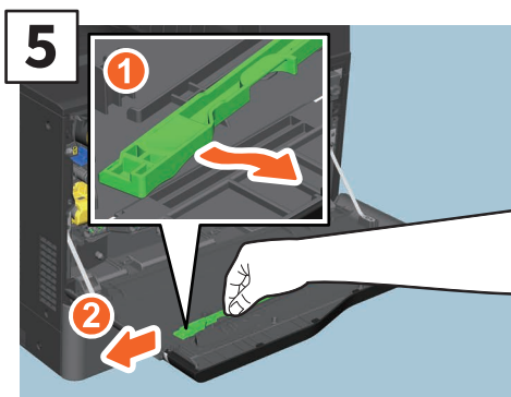
5 Haal de groene reiniger aan de binnkant van het deksel eruit.
